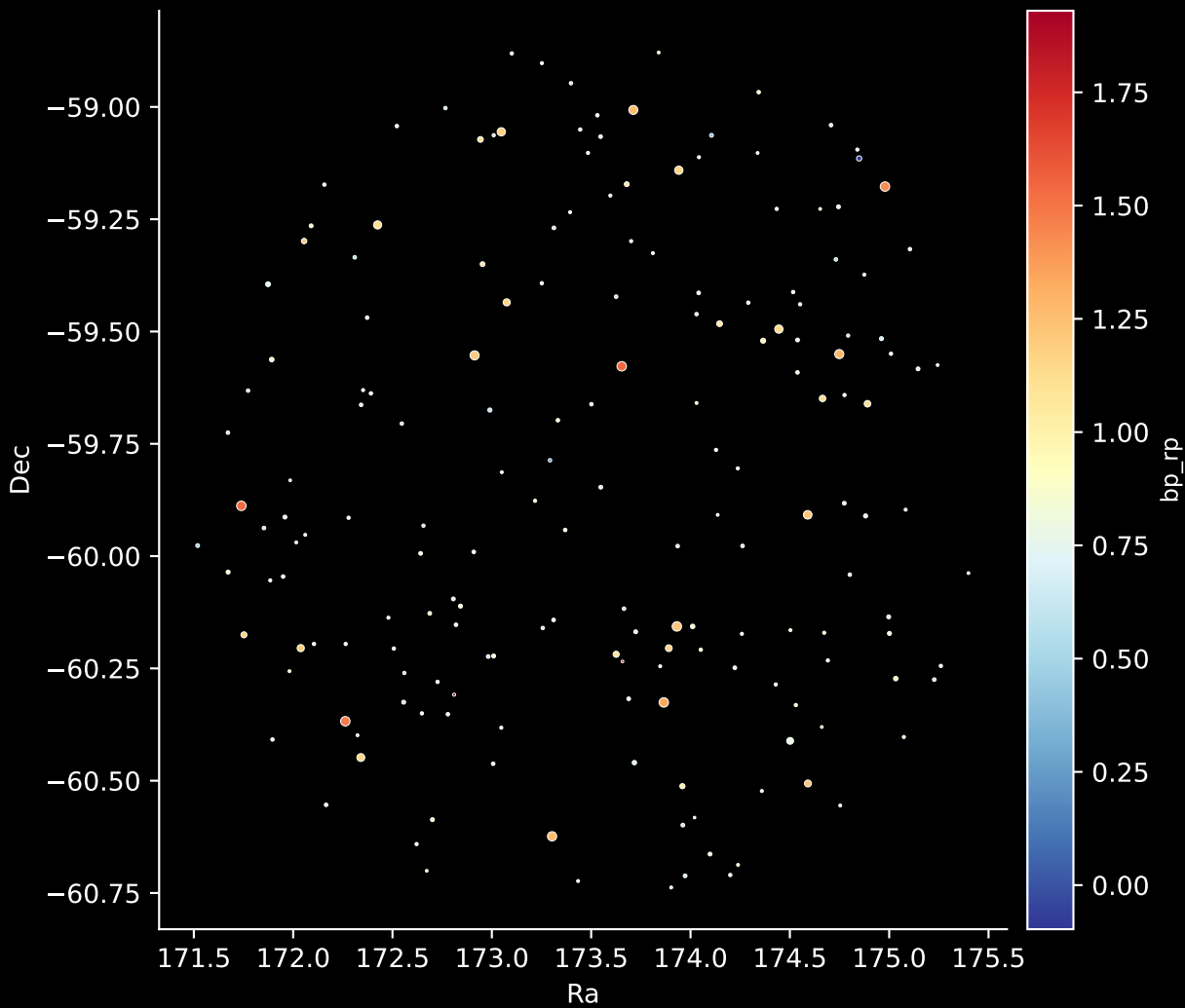
GALAH DR4 Field: [7182] Stars: 179
