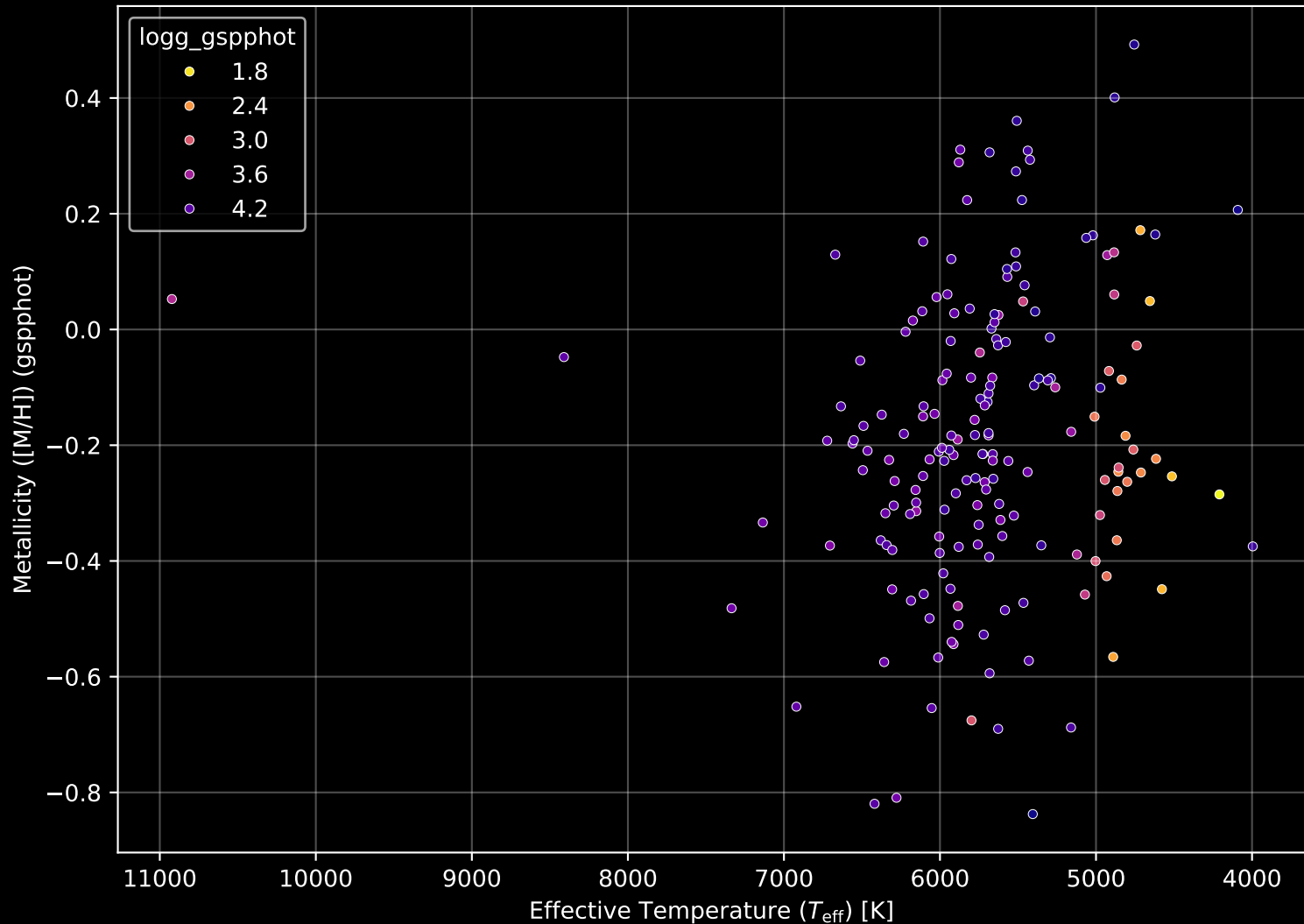
GALAH DR4 Field: [7182] Stellar Population Parameters (n= 179)
